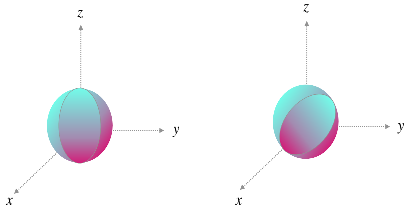
شکل ۲: سمت راست: تغییر کره بلوخ تحت تاثیر کانال بیت - برگردان، سمت راست: تغییر کره بلوخ تحت تاثیر کانال فازبرگردان
